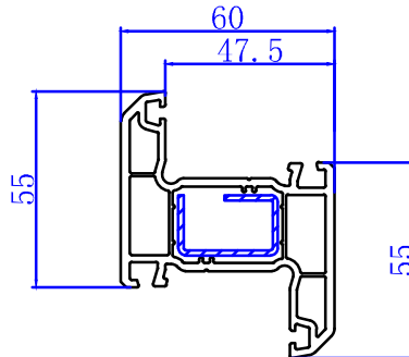
60 Outward Door Sash 311300
