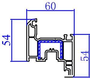
60 Inward Window Sash 310200
