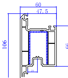
60 Outward Door Sash 311300
