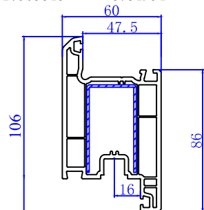
60 Inward Door Sash 310600
