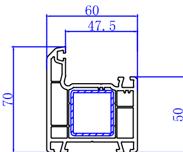
60 Door Frame 310500
